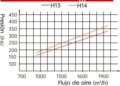
Diagrama de flujo de aire y resistencia 644*644*150
